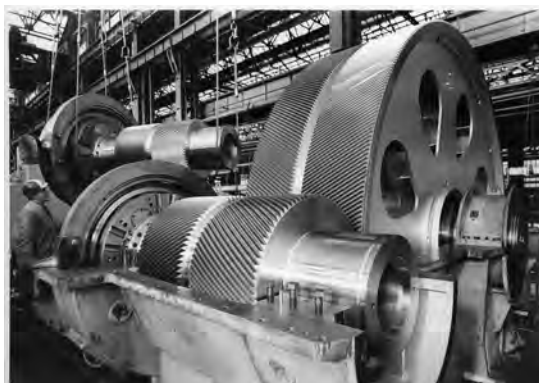
شکل ۲۶ - جعبه دنده یک شناور بزرگ
