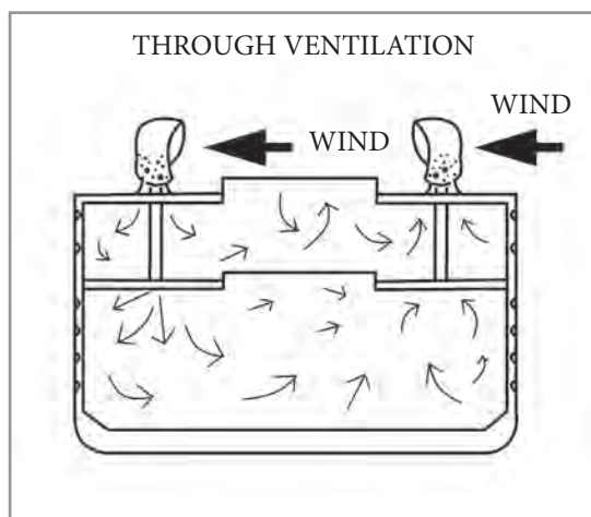
شکل ۵- تهویه سراسری
