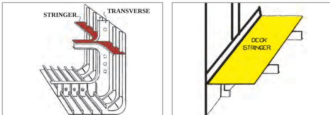
شکل ۲۸- محکم کننده عرضی
