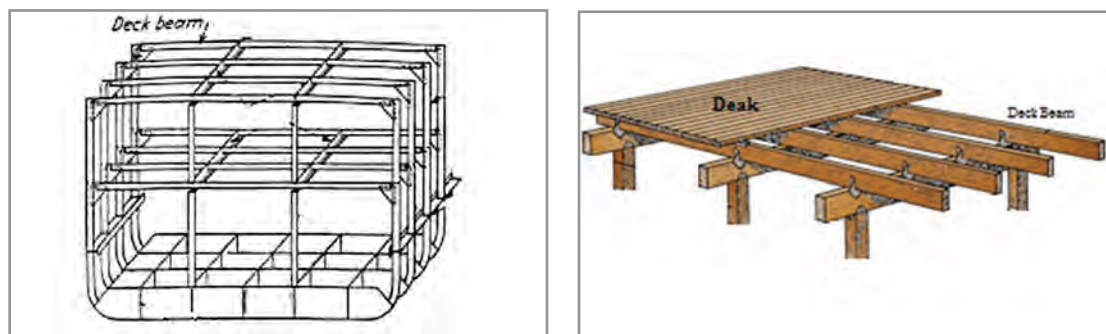
شکل ۲۹- تیرچه سقفی
