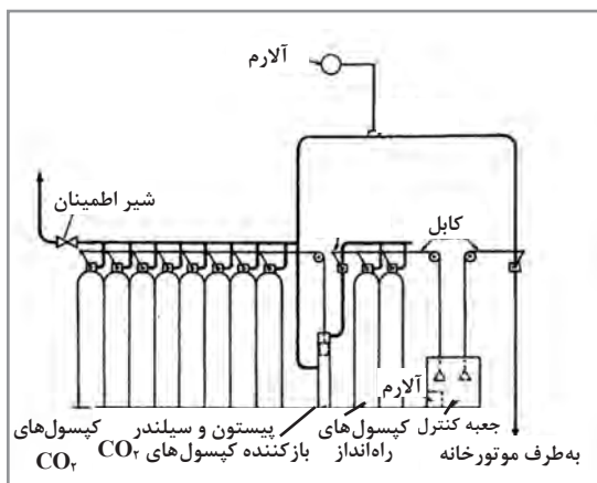
شکل ۳۸- سامانه اطفای حریق \text{CO}_2
